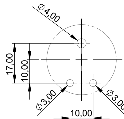
Bohrschablone M. 1:1
